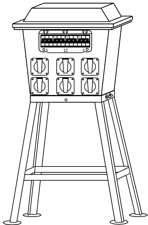
Linker aanzicht
