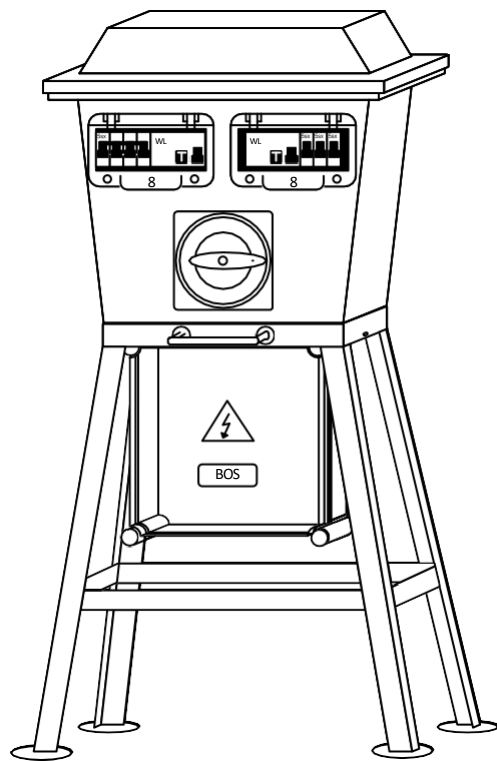
Vooranzicht
