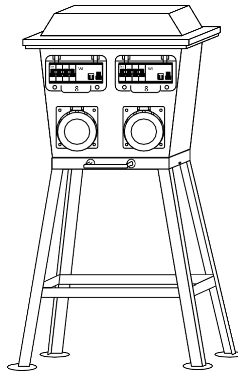
Achteraanzicht
