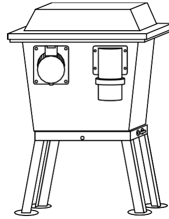
Achteraanzicht
